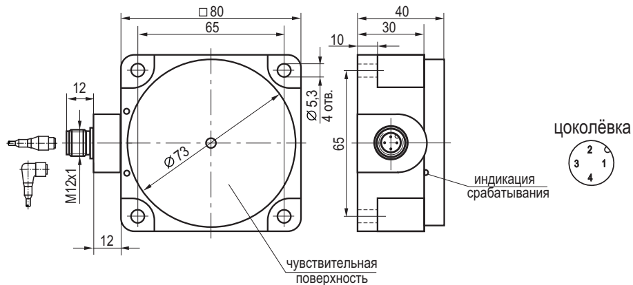
Габаритный чертеж
